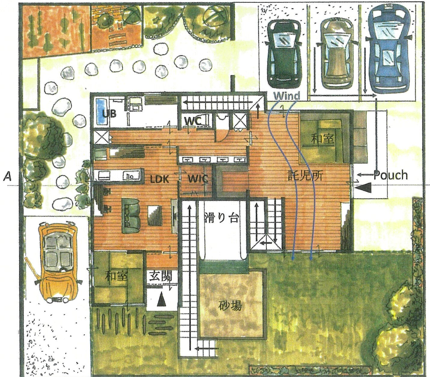
配置図兼一階平面図
