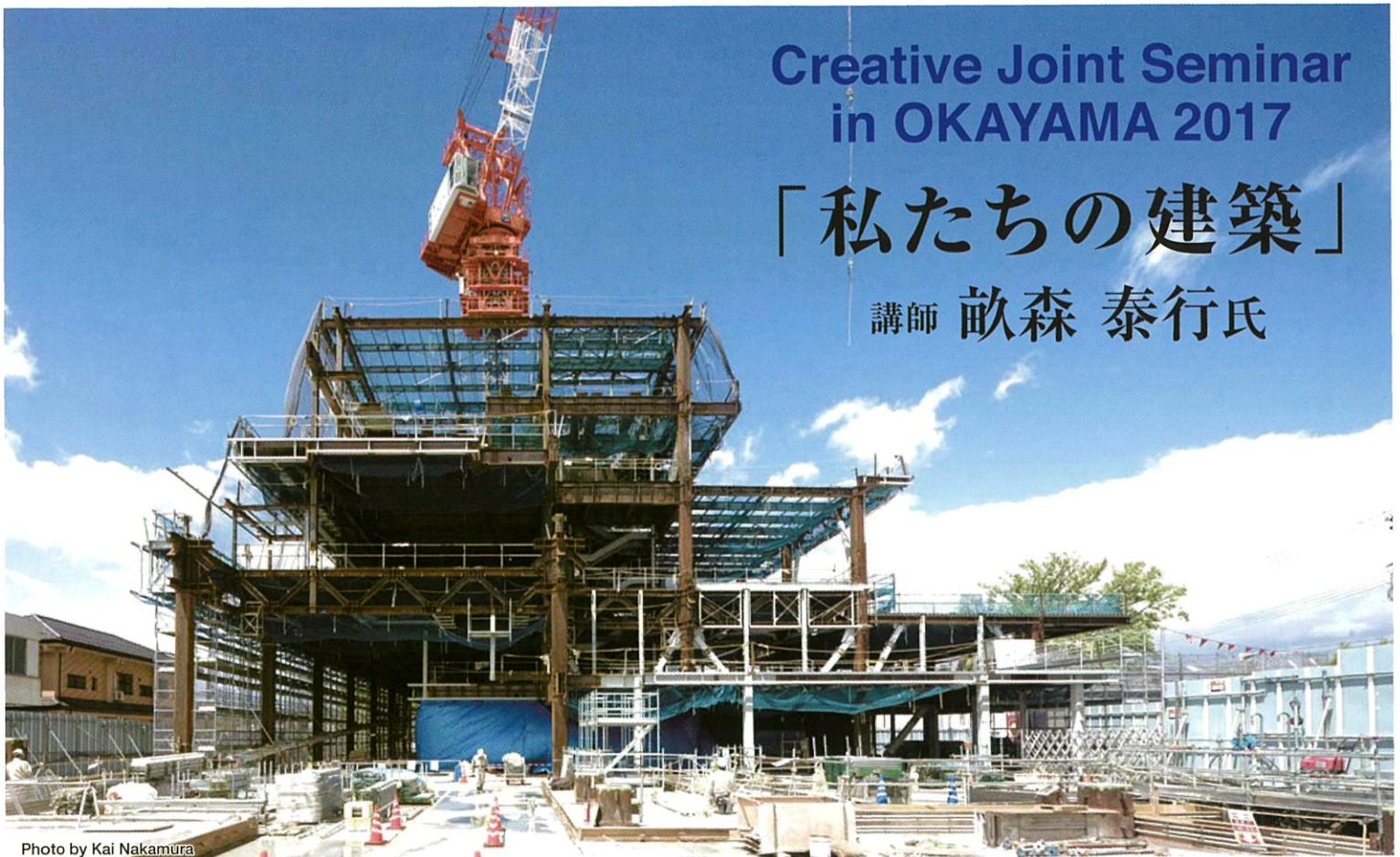
須賀川市 市民交流センター tette(共同設計:石本建築事務所)
